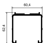
CASSONETTO HEAD BOX CAISSON
