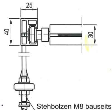
Montage mit Schwertkonsole
