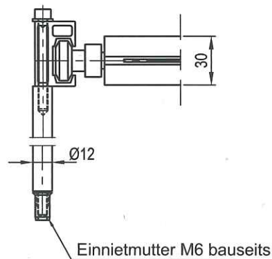
Montage mit Abstandhalter Ø12
