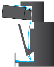
Geschlossenes Dach
