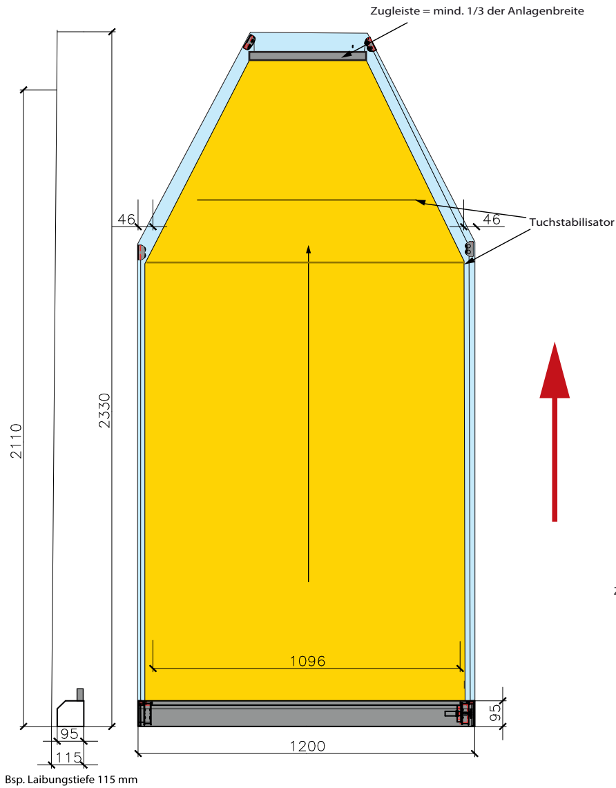
Bsp. ausgefahrene Schrägmarkise UNO 95.2 am Mustermaß Breite 1200 mm x Höhe 2330 mm
