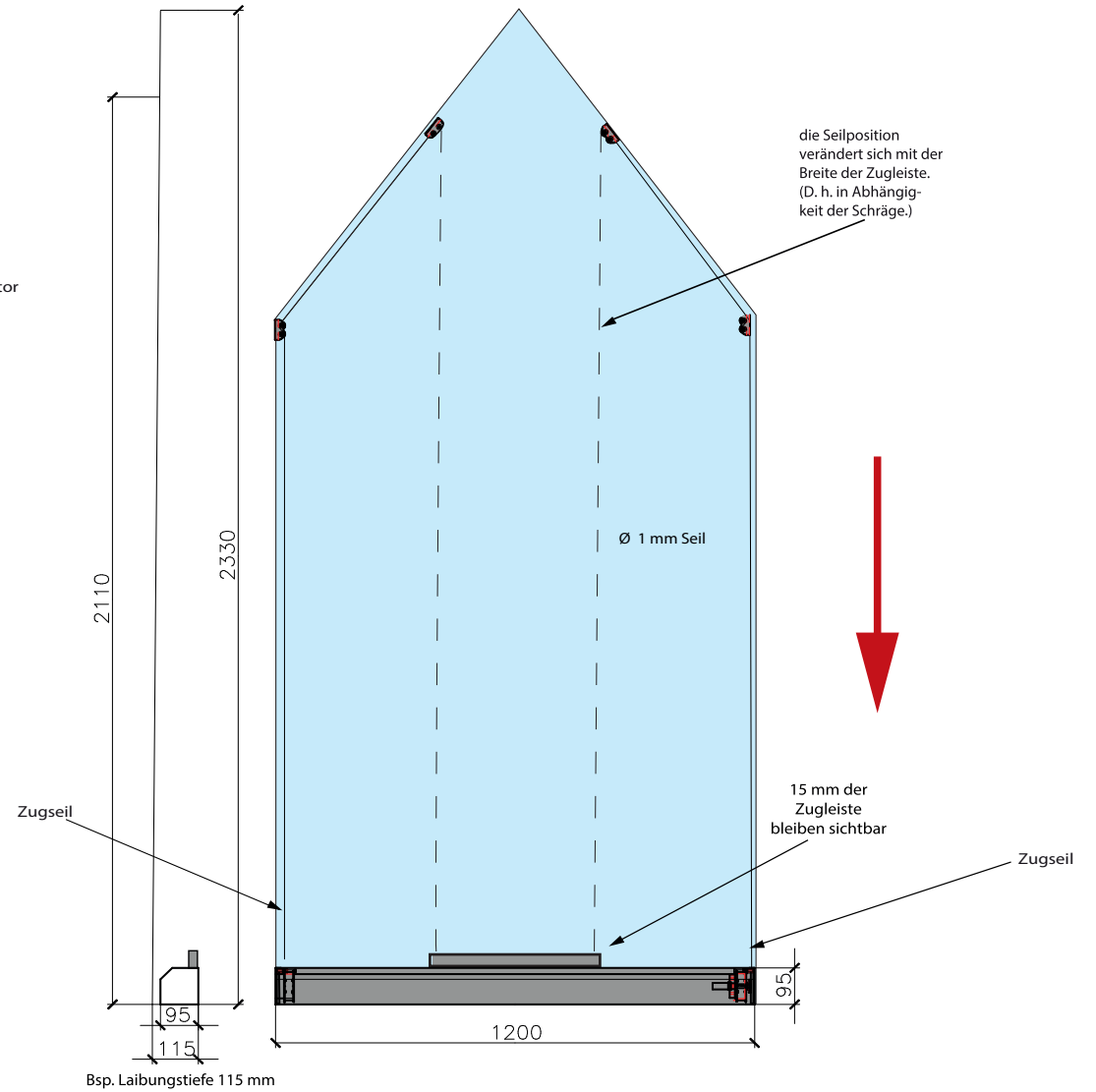
Bsp. eingefahrene Giebelmarkise UNO 95.2 am Mustermaß Breite 1200 x Höhe 2330 mm
