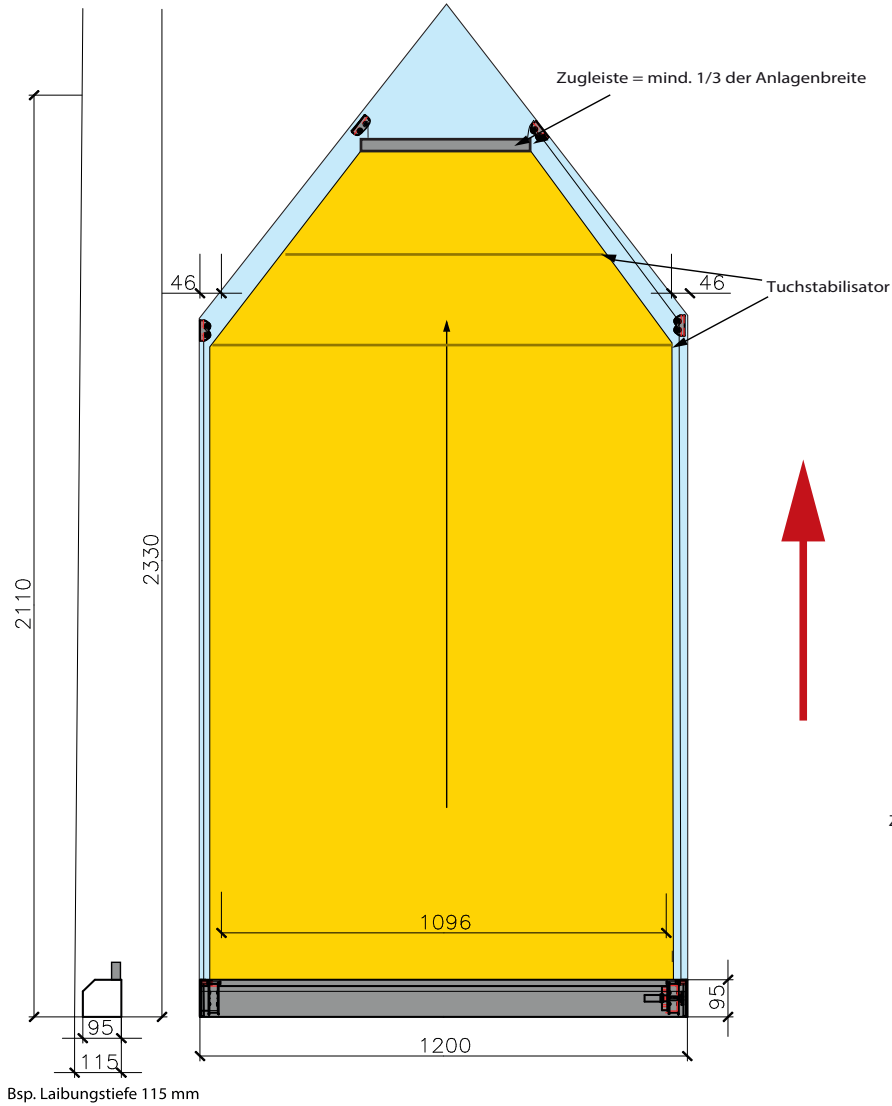
Bsp. ausgefahrene Giebelmarkise UNO 95.2 am Mustermaß Breite 1200 x Höhe 2330 mm
