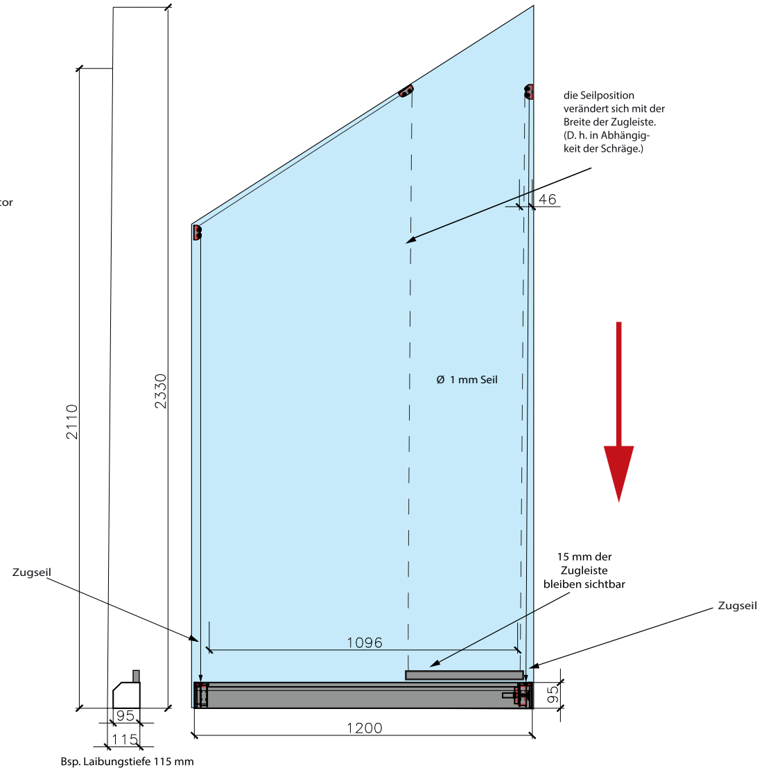
Bsp. eingefahrene Schrägmarkise UNO 95.2 am Mustermaß 1200 x 2330 mm
