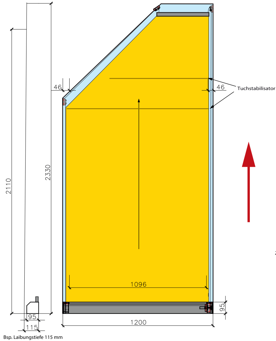
Bsp. ausgefahrene Schrägmarkise UNO 95.2 am Mustermaß Breite 1200 mm x Höhe 2330 mm
